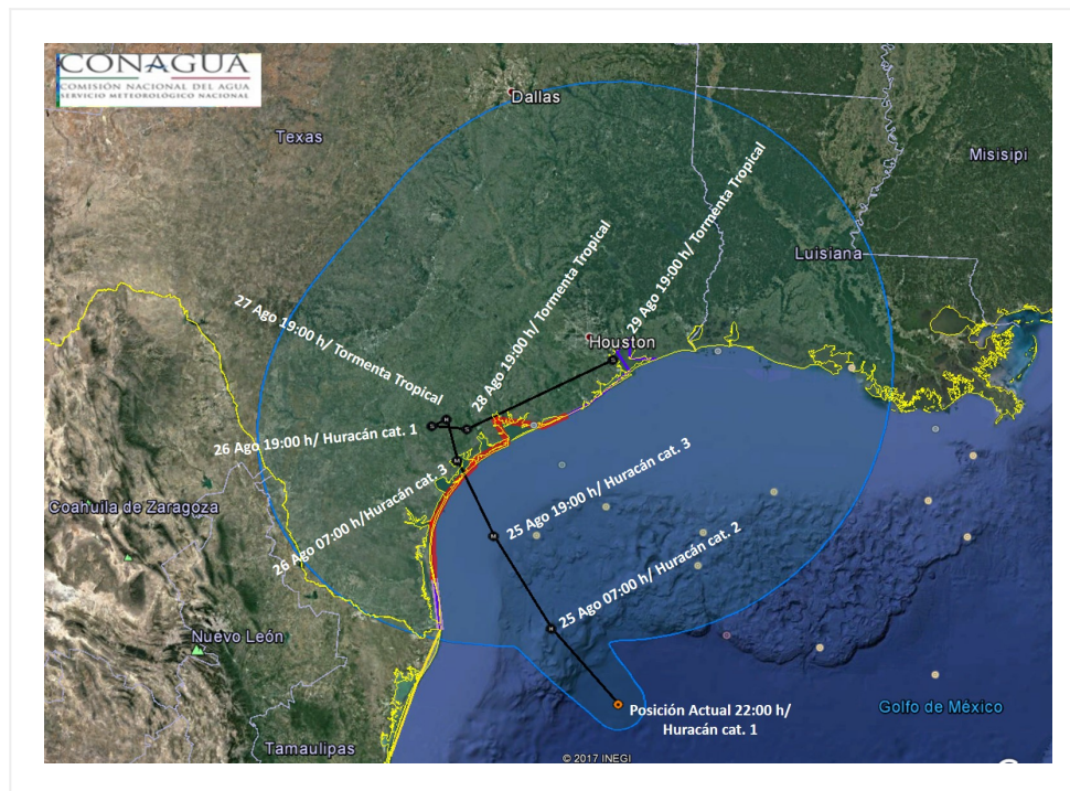
Trayectoria pronóstico del Huracán cat. 1 "HARVEY"
